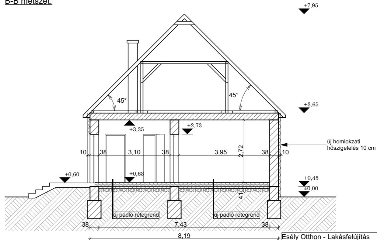
B-B metszet:
