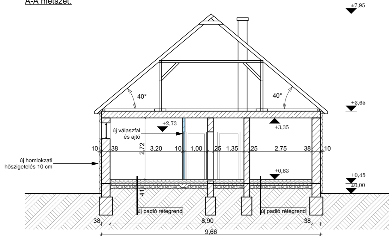
A-A metszet:
